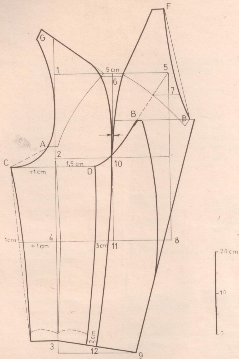
Слика 8.37. Конструкција раглан рукава из три дела
